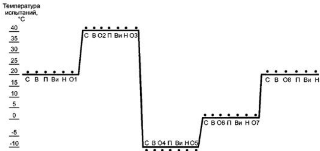
Рисунок 11 - Предлагаемая последовательность испытаний по А.5.3.1, совмещенных с А.5.3.2 (температурные испытания в диапазоне от минус 10 °С до плюс 40 °С)
