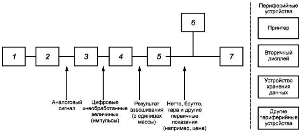
Рисунок 1 - Функциональная блок-схема весов и состав типичных модулей в соответствии с Т.2.2 и 3.10.2
