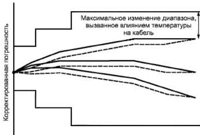
Рисунок 12 - Изменение диапазона из-за влияния температуры на кабель
