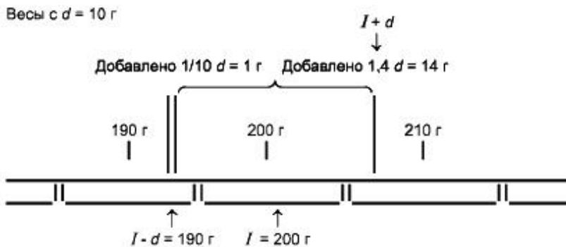
Рисунок 10 - Реагирование весов на дополнительные гири
