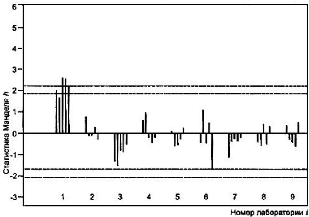
Рисунок В.7 - Титрование креозотового масла. Значения статистики межлабораторной совместимости Манделя h , сгруппированные по лабораториям
